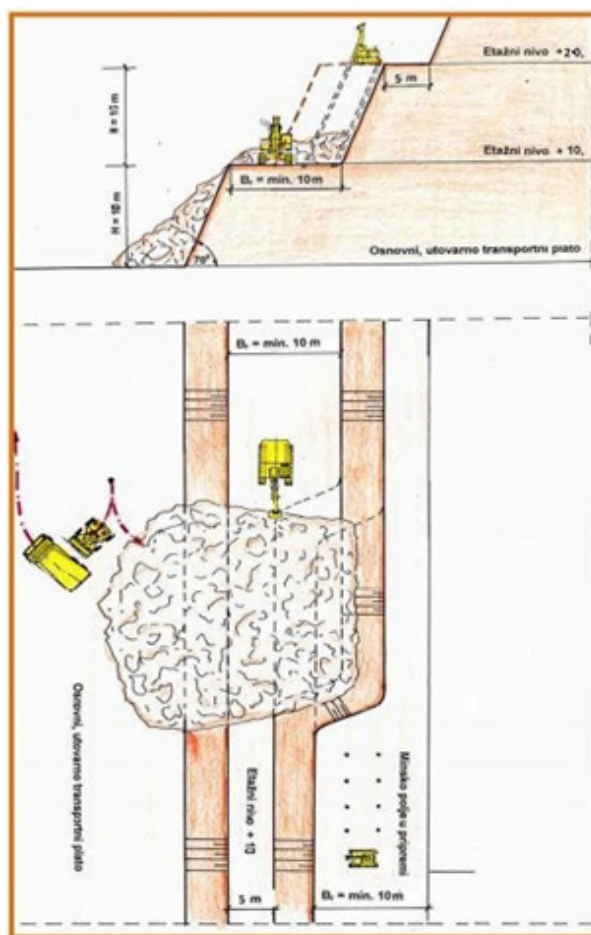
Slika br. 7. Tehnološka šema bušenja i miniranja
