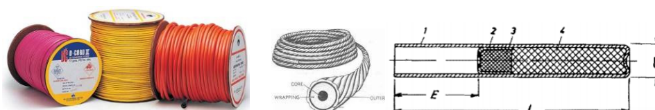
Slika br. 12 Izgled detonirajućeg, sporogorećeg štapina i detonirajuće kapisle
