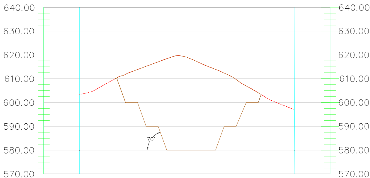
Slika br. 20 Visinska podjela površinskog kopa „Kruševice II“ – Profil br. 11-11´
