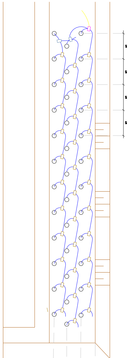
Slika br. 16 Višeredna šema Iniciranja minskih bušotina Nonel sistemom
