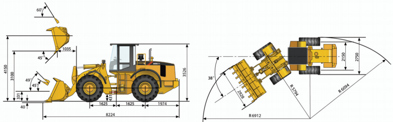
Slika br. 26 Konstruktivne karakteristike utovarača LiuGong 856
