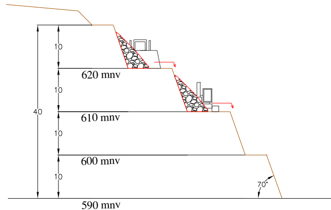
Slika br. 28 Gravitacijsko obaranje materijala
