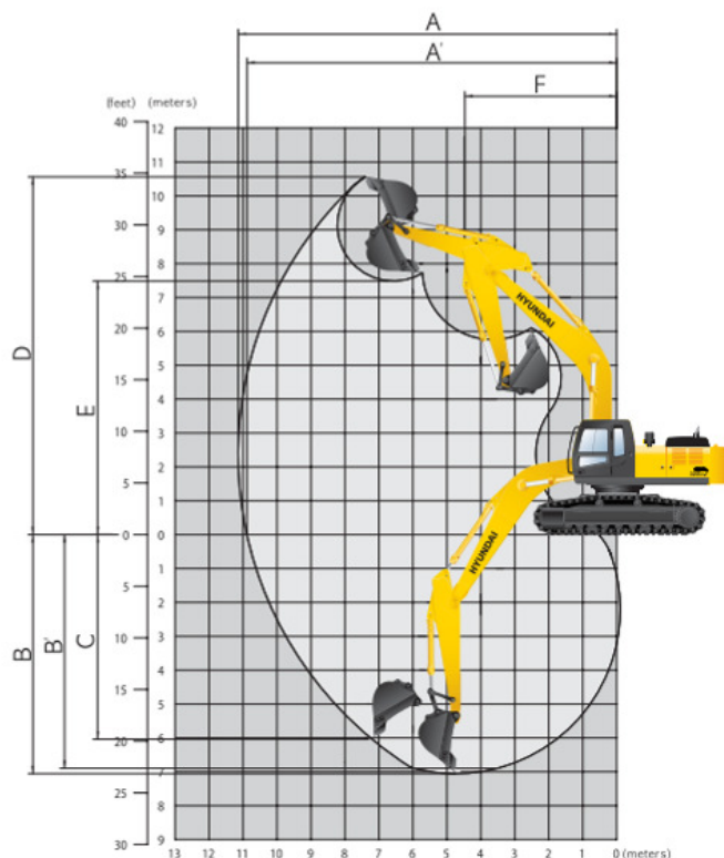
Slika br. 23 Tehničke karakteristike bagera HYUNDAI R320LC-7
