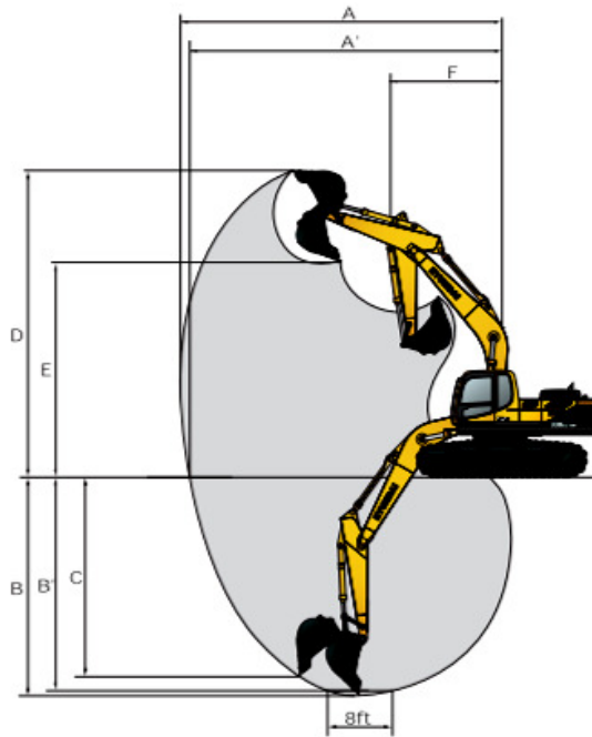
Slika br. 22 Tehničke karakteristike bagera HYUNDAI 330 LC-95
