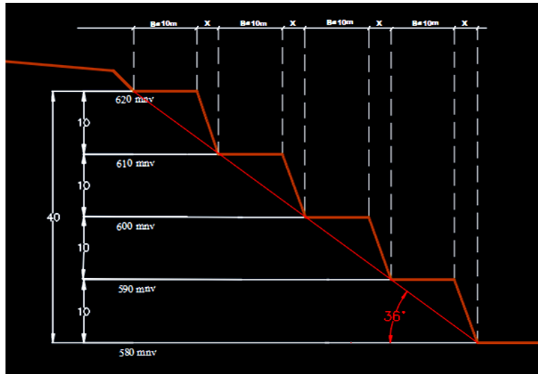
Slika br. 4. Ugao nagiba završne kosine za minimalnu širinu berme B=10\text{ m}
