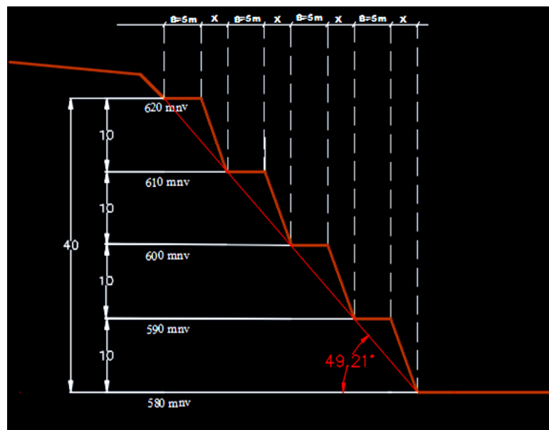
Slika br. 3. Ugao nagiba završne kosine za minimalnu širinu berme B=5 \text{ m}
