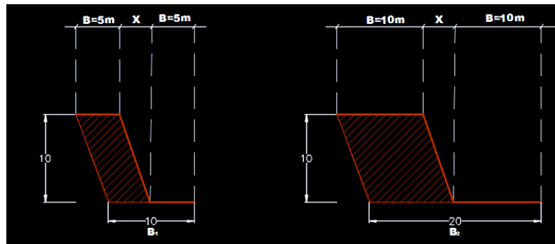
Slika br. 1. Širina otkopnog bloka za korak napredovanja od 5 i 10 m
