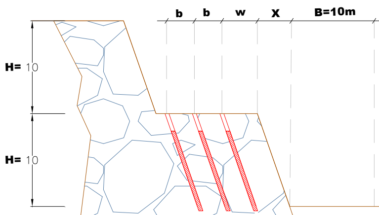
Slika br. 9 Konstrukcija minskog punjenja za etažu visine H=10 m
