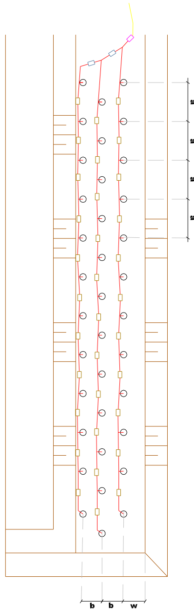
Slika br. 15 Višeredna šema iniciranja minskih bušotina det. stapin-udarna patrona
