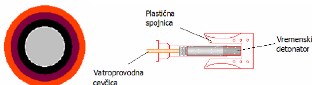
Slika br.11 Poprečni presijek Nonel vatroprovodne cijevčice i izgled Nonel konektora
