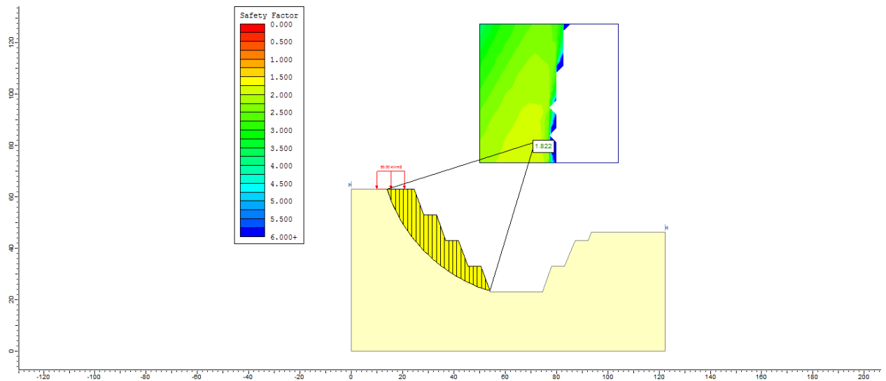
Slika br. 5. Analiza geološkog profila po numeričkoj metodi Janbu koja je pokazala najmanji koeficijent stabilnosti lijeve strane F_s=1,822
