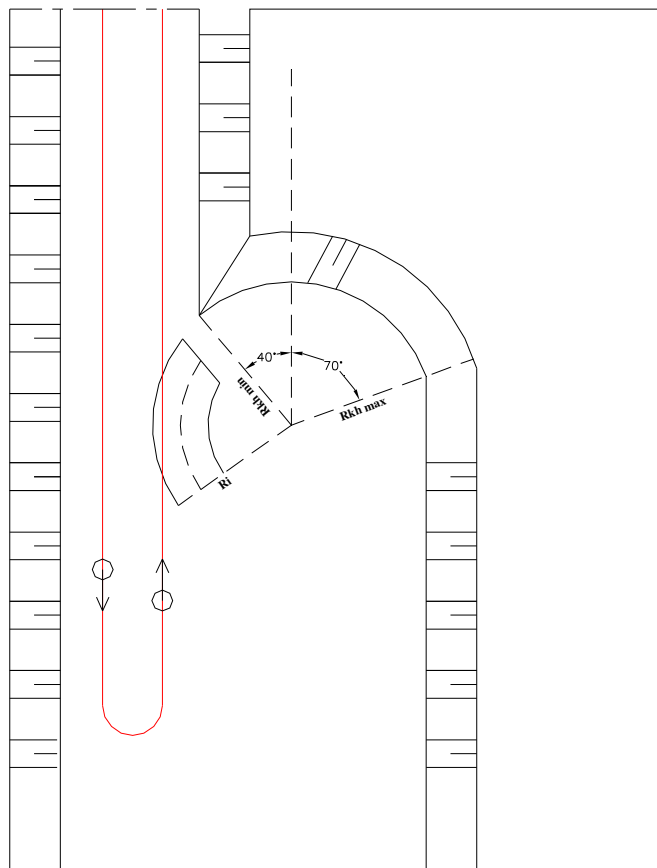
Slika br. 24. Tehnološka šema rada bagera
