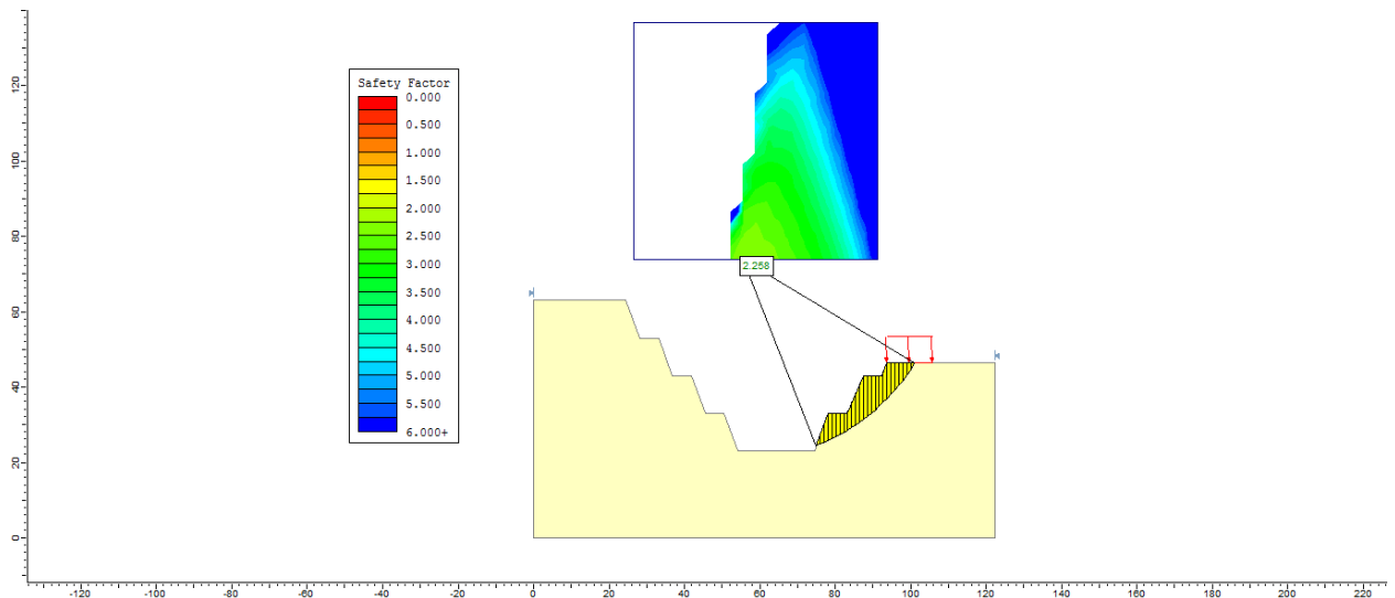
Slika br. 6. Analiza geološkog profila po numeričkoj metodi Janbu koja je pokazala najmanji koeficijent stabilnosti desne strane F_s=2,258
