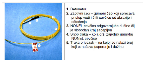
Slika br. 10 Izgled Nonel sistema detonatora
