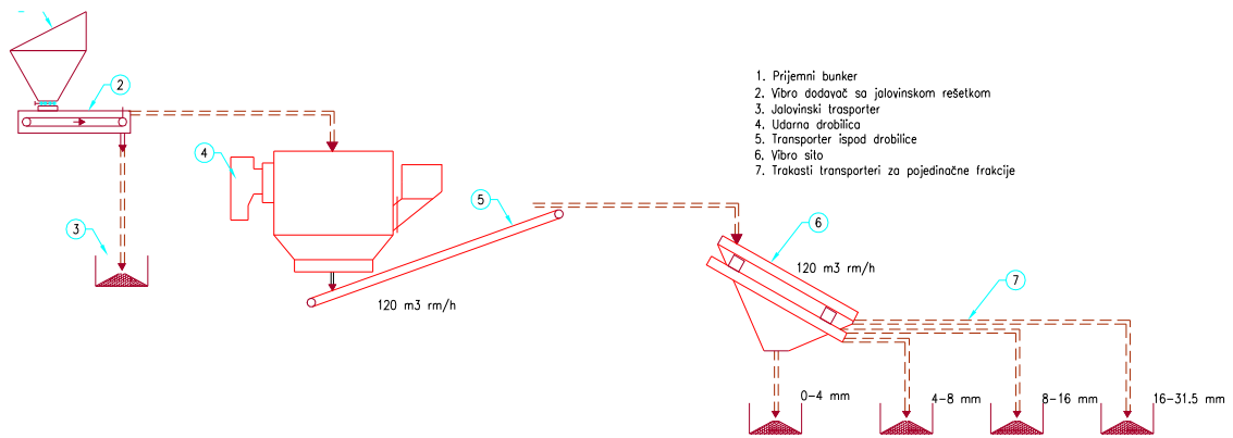
Slika br. 32 Tehnološka šema rada postrojenja
