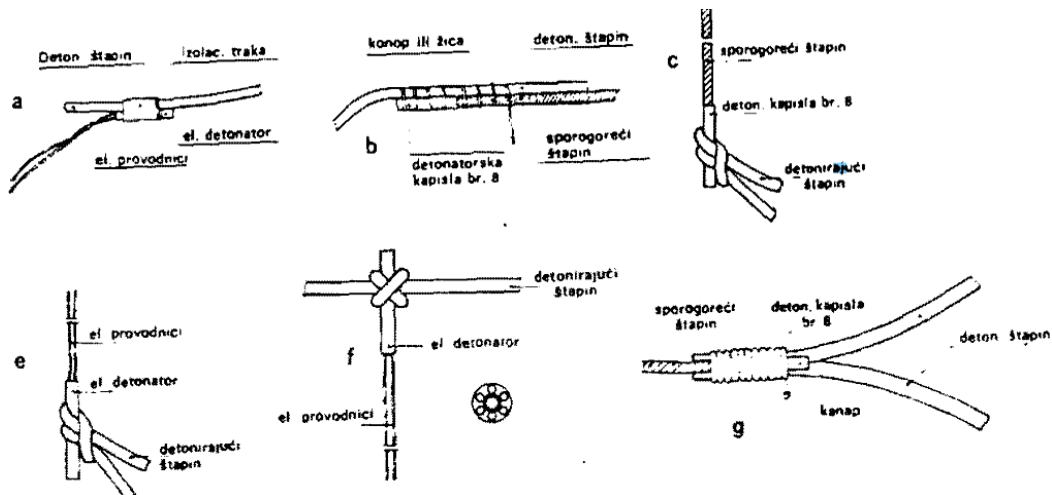
Slika br. 13 Prikaz grananja i vezivanja detonirajućeg štapina
