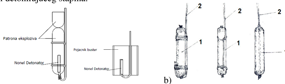
Slika br. 14 Podešavanje udarne patrone, pojačivača i prikaz povezivanja udarne patrone
