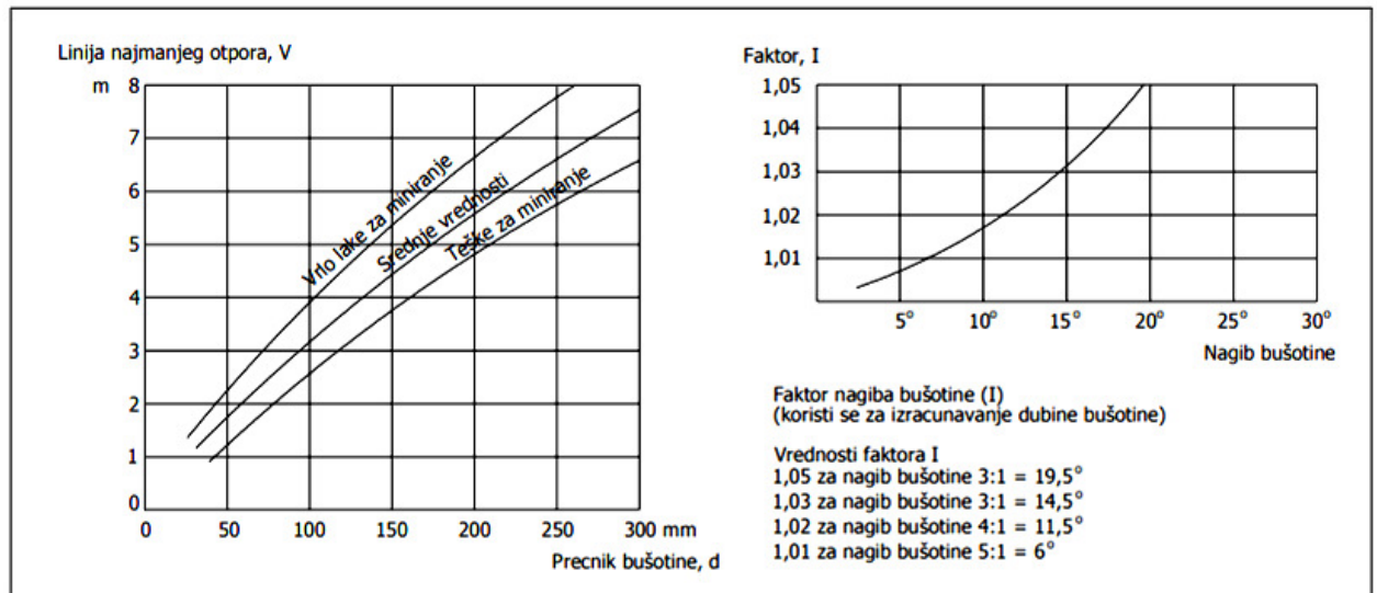
Slika br. 8 Odnos prečnika bušotine i linije najmanjeg otpora
