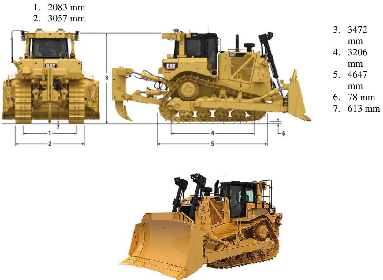
Slika br. 25 Konstruktivne karakteristike buldozera Caterpillar D8L
