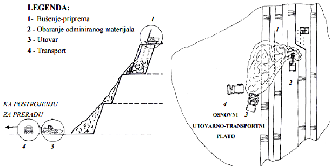
Slika br. 19. Principijelna šema tehnološkog procesa dobijanja krečnjaka
