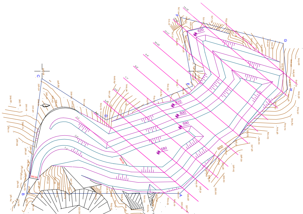
Slika br. 21 Završna kontura površinskog kopa „Kruševice I“
