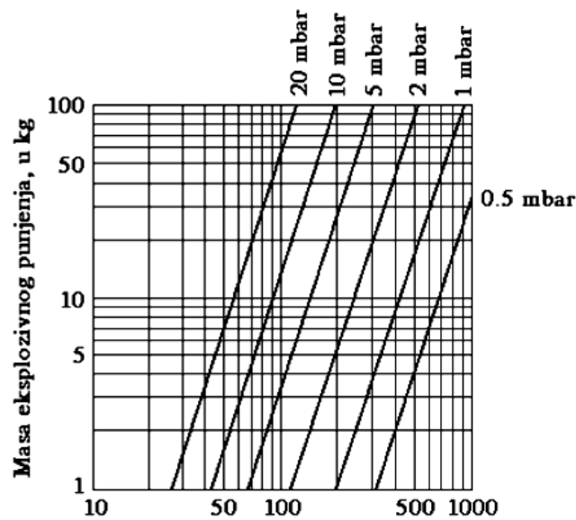
Slika br. 18 Dijagram za određivanje vazdušnog nadpritiska u funkciji kolicine eksploziva
