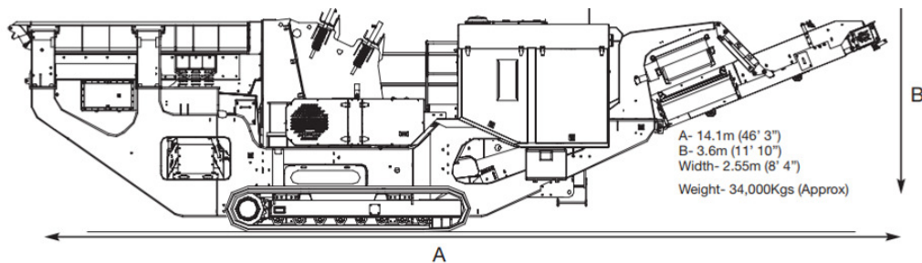
Slika br. 30 Dimenzije mobilnog drobiličnog postrojenja Terex Finlay I-1310
