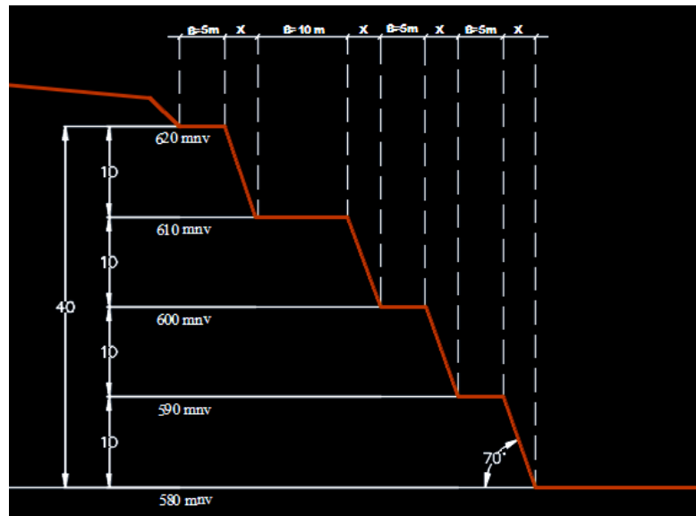
Slika br. 2. Konstruktivni parametri površinskog kopa „Kruševice I“
