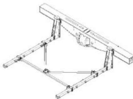
Šema nosača baterija sa ukrućenjem
