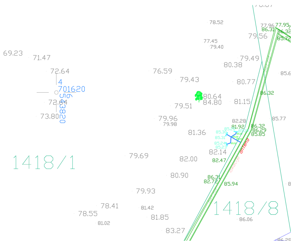
Slika 2.4. Prikaz katastarskih parcela (sa ucrtanim planiranim projektom)
