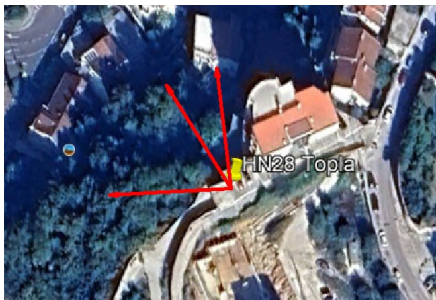
Slika 4.1. Pozicija antena sa ucrtanim pravcima i graničnim zonama
