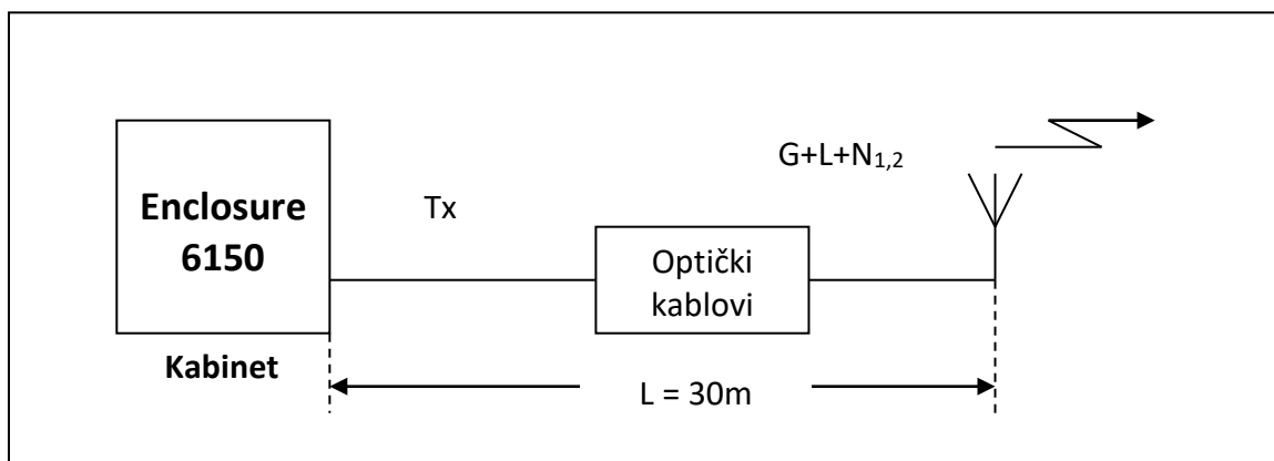
Skica: Proračun efektivne izračene snage
