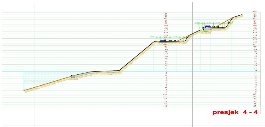
Slika 3.3. Profil kroz plažu i parking
