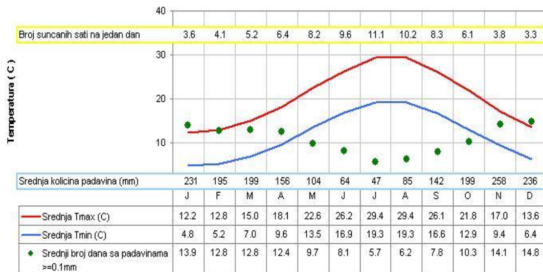
Slika 6.5.1. Dijagram najznačajnijih prosječnih klimatskih parametara za opštinu Herceg Novi
