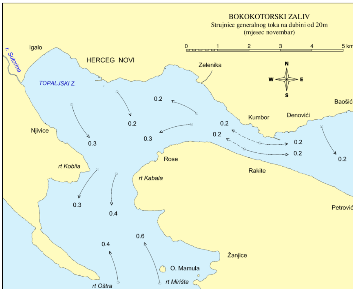
Slika 6.8.2. Strujnice generalnog toka na dubini od 20 m za mjesec novembar (brzine u čvorovima) (prema: Vodopija i sar., 1976)
